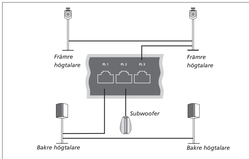
Exempel på högtalarinstallation.
