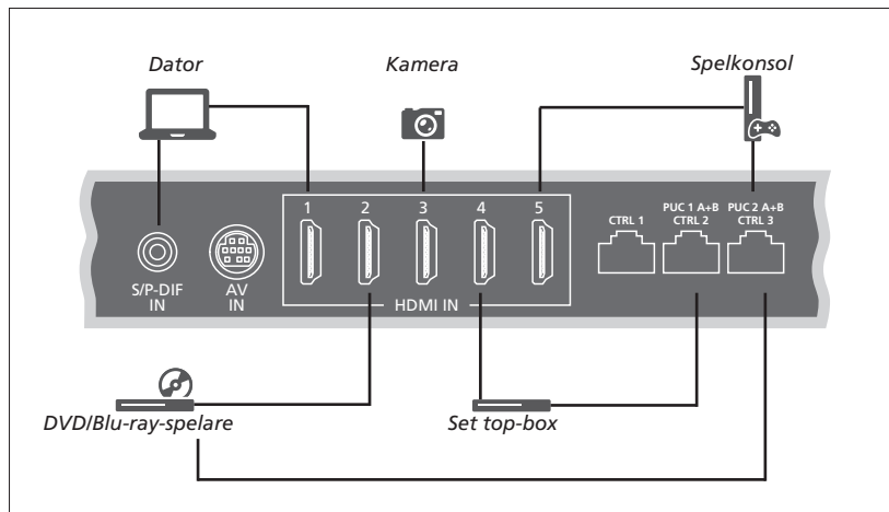
Exempel på anslutna digitala källor.
