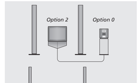
BeoCenter 1 och ett audiosystem i ett rum – alla högtalarna är anslutna till BeoCenter 1.
